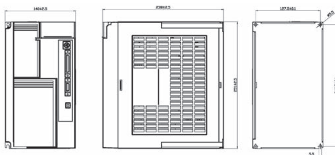
TSTG 200D / 300D 尺寸图
